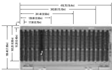
GHP-2020 20xISA Slot
